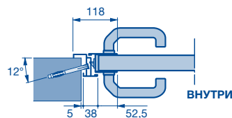
Тип профиля 2 (дверь открывается наружу)
